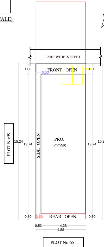
SITE PLAN SCALE : 1:100
