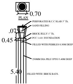
PER SECTION
