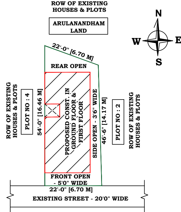
SITE PLAN:
