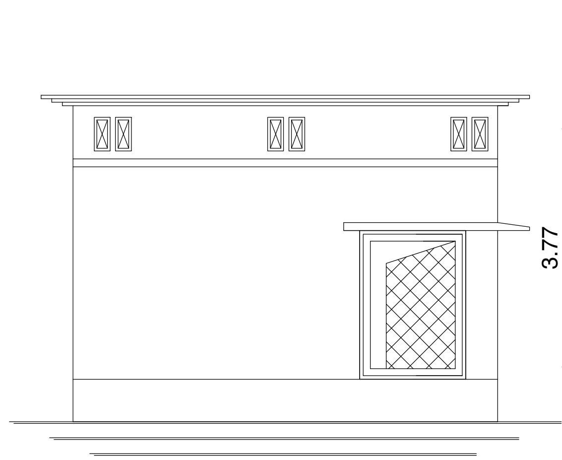
ELEVATION
