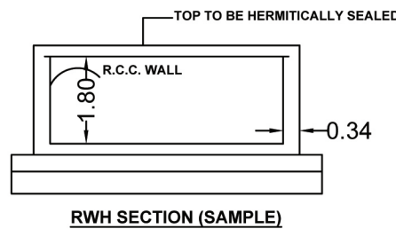
RWTH_CAPACITY_L=5000LTRS
