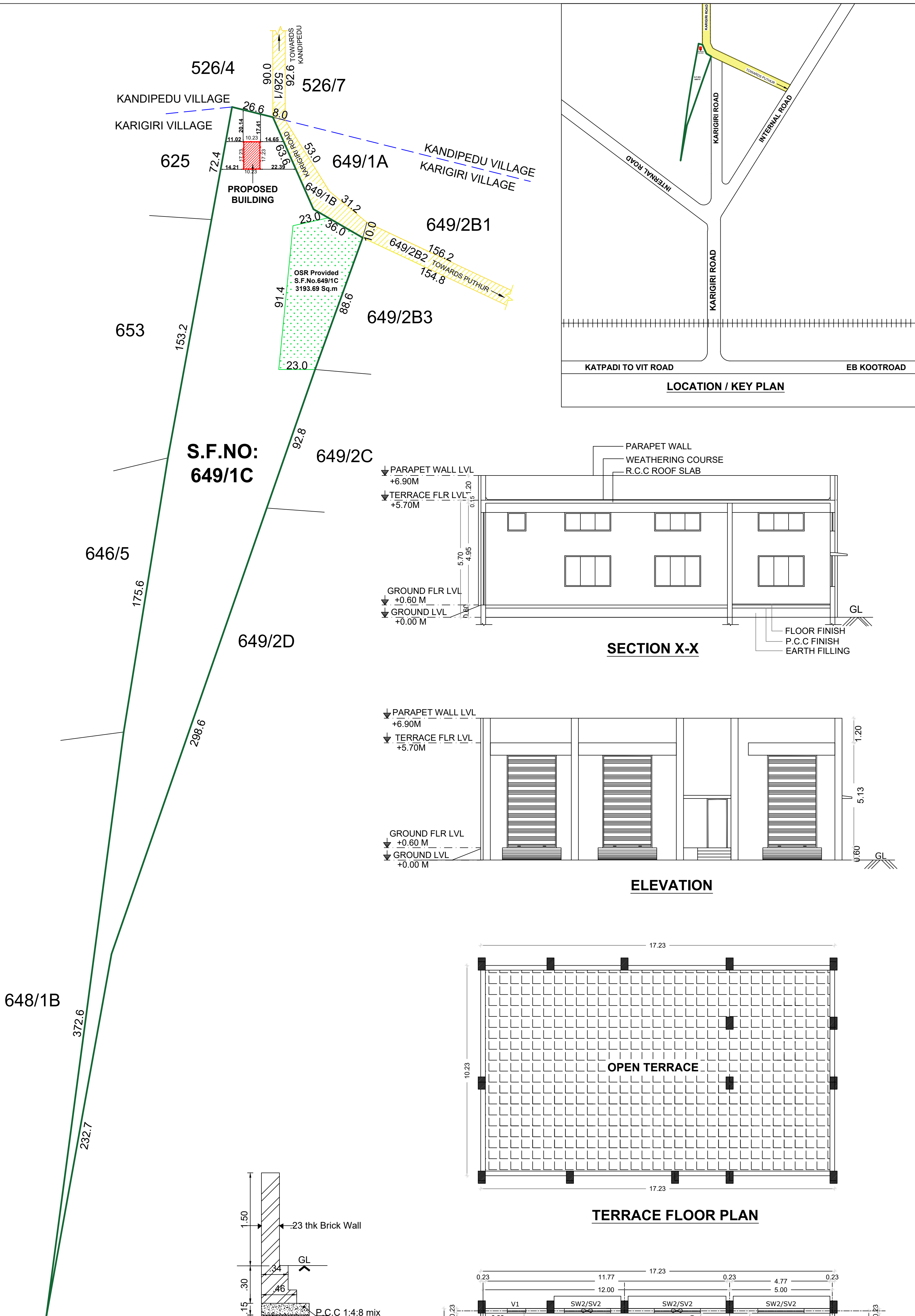
SITE PLAN 1:1000
