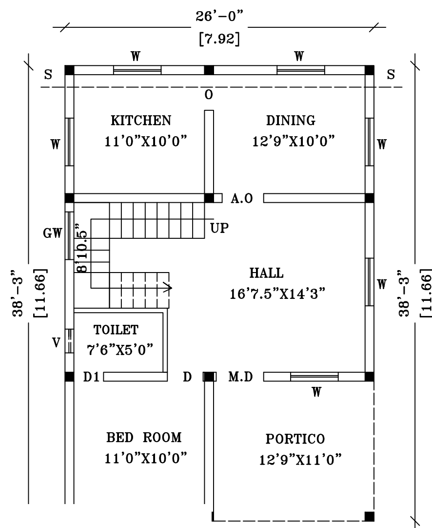
'LOOR PLAN
