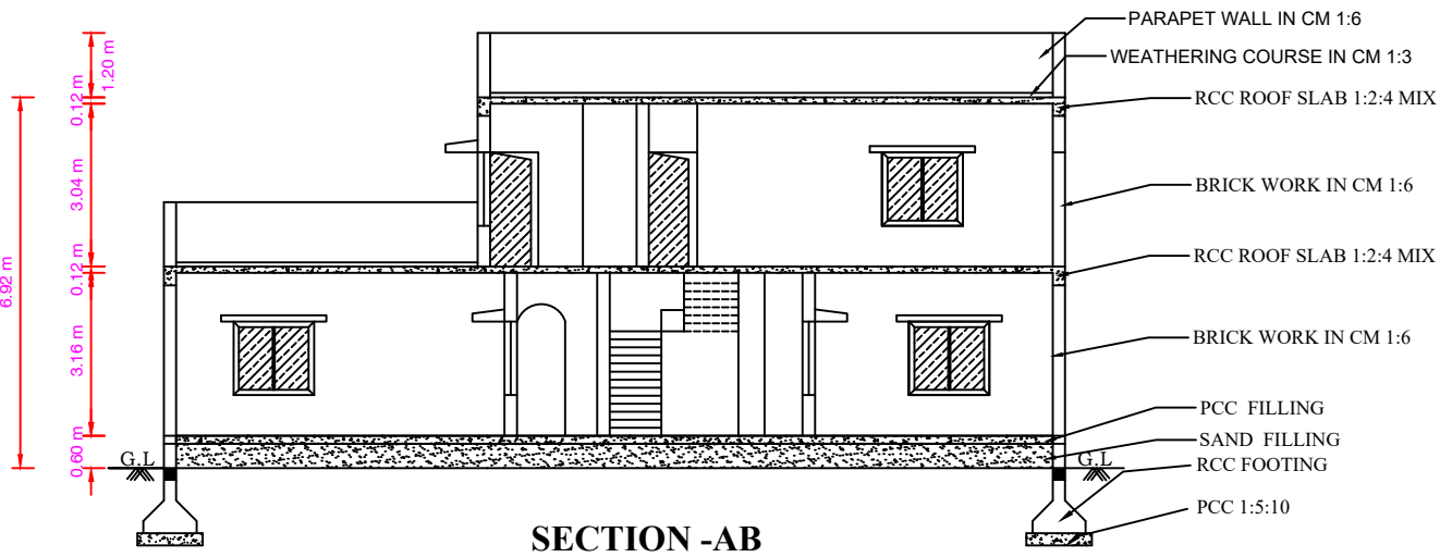
SECTION -AB
