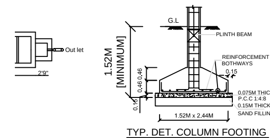
TYP. DET. COLUMN FOOTING
