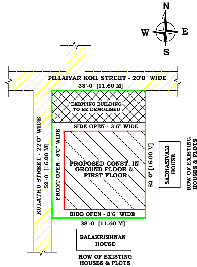
SITE PLAN:
