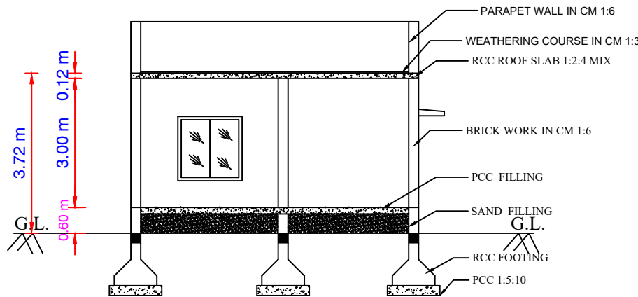
SECTION - AB
