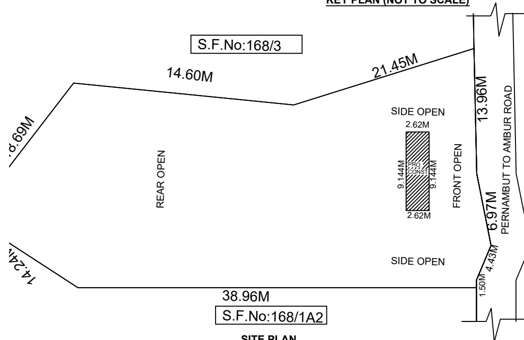
SITE PLAN SCALE 1:400
