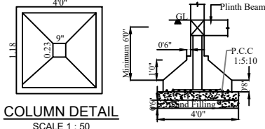
COLUMN DETAIL SCALE: 1:50
