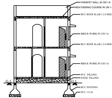
SECTION - AB
