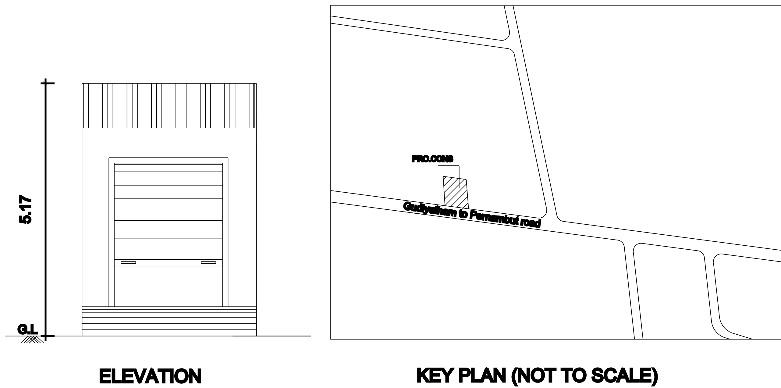
ELEVATION
