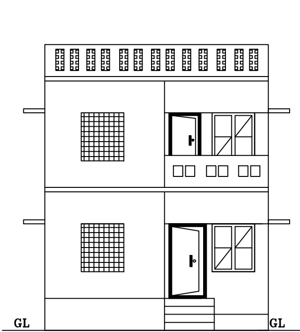
ELEVATION
