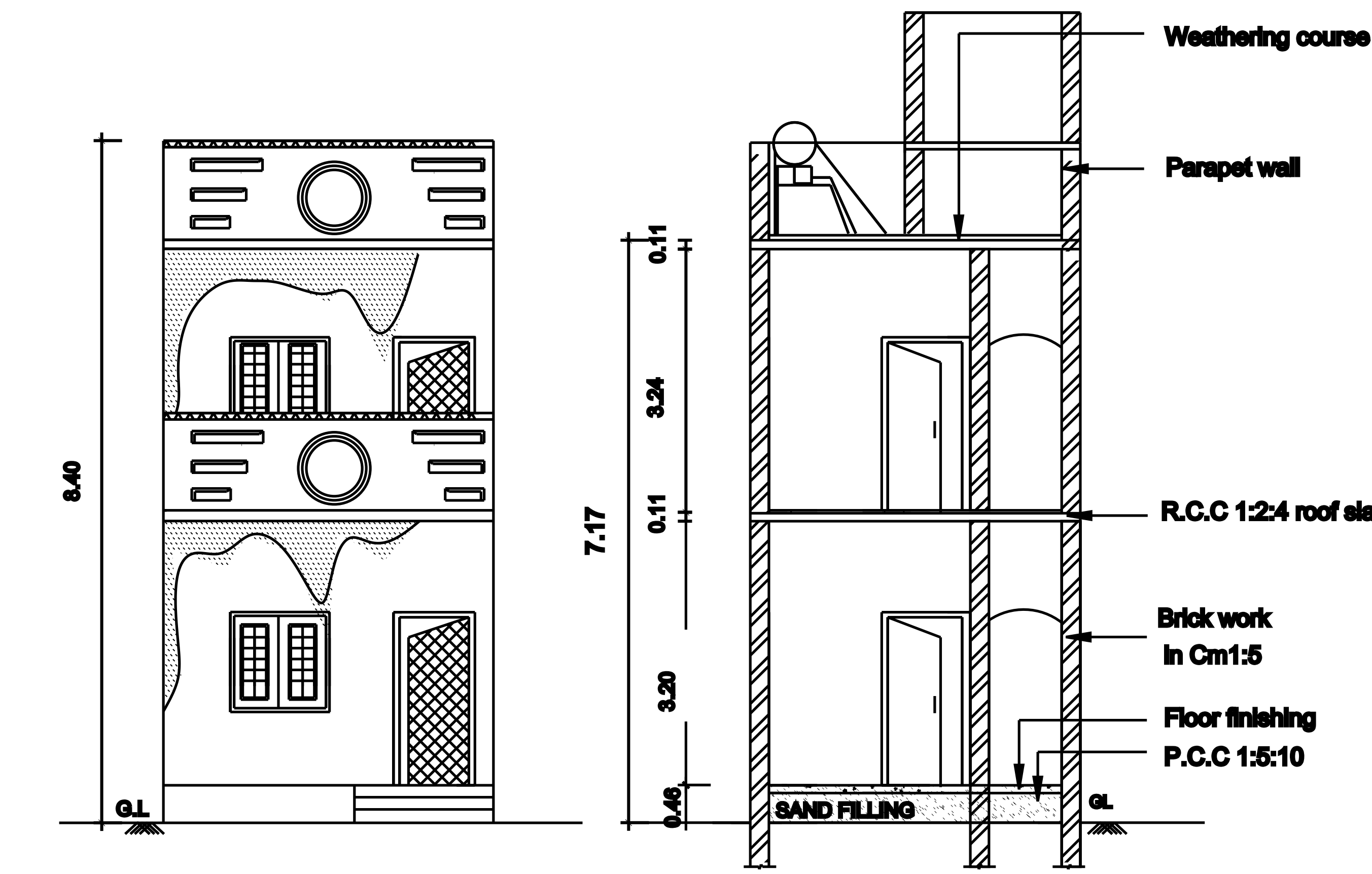
ELEVATION
