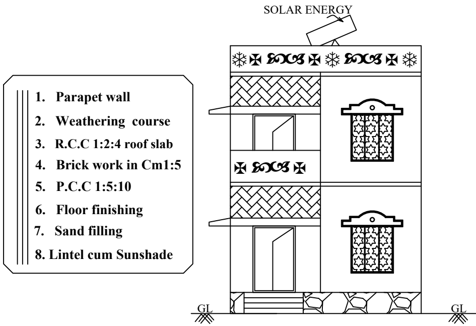
ELEVATION
