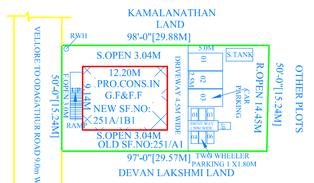
SITE PLAN SCALE-1:400
