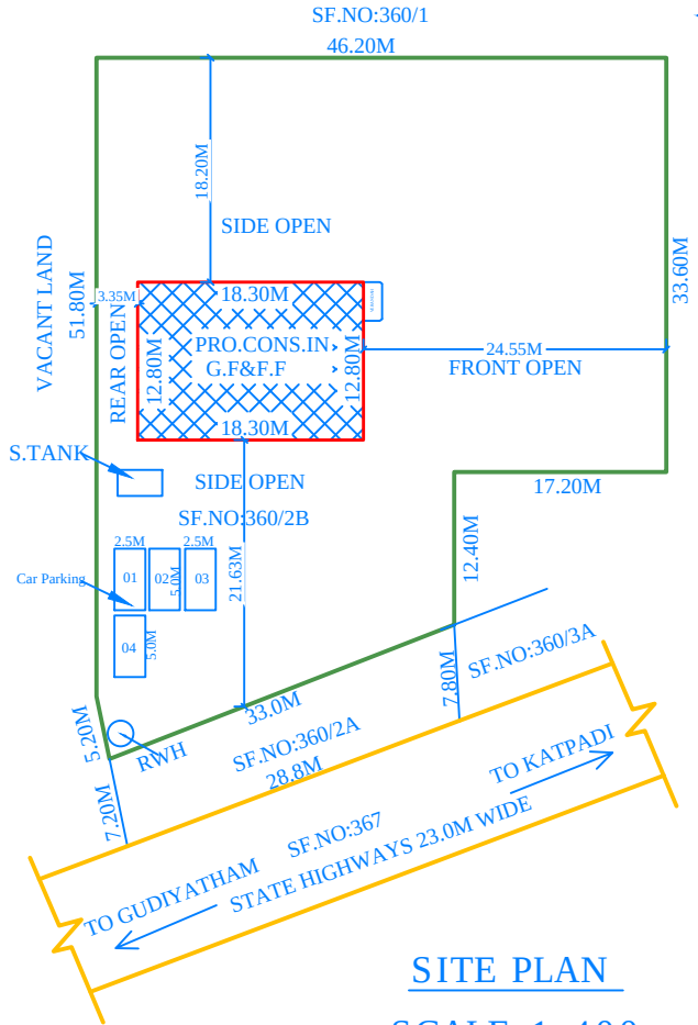
SCALE-1:400
