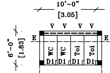
TOILET PLAN
