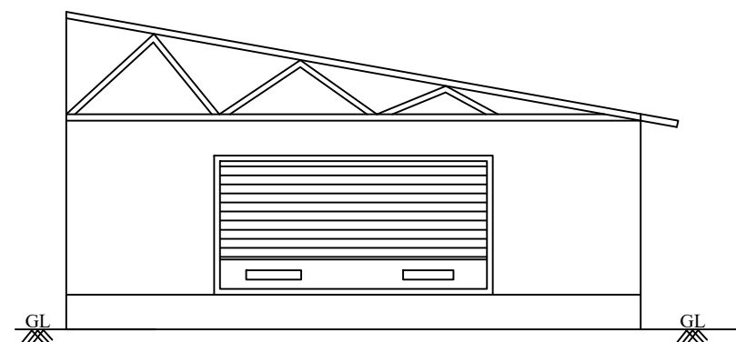
ELEVATION
