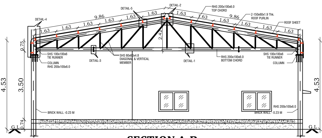
SECTION A-B
