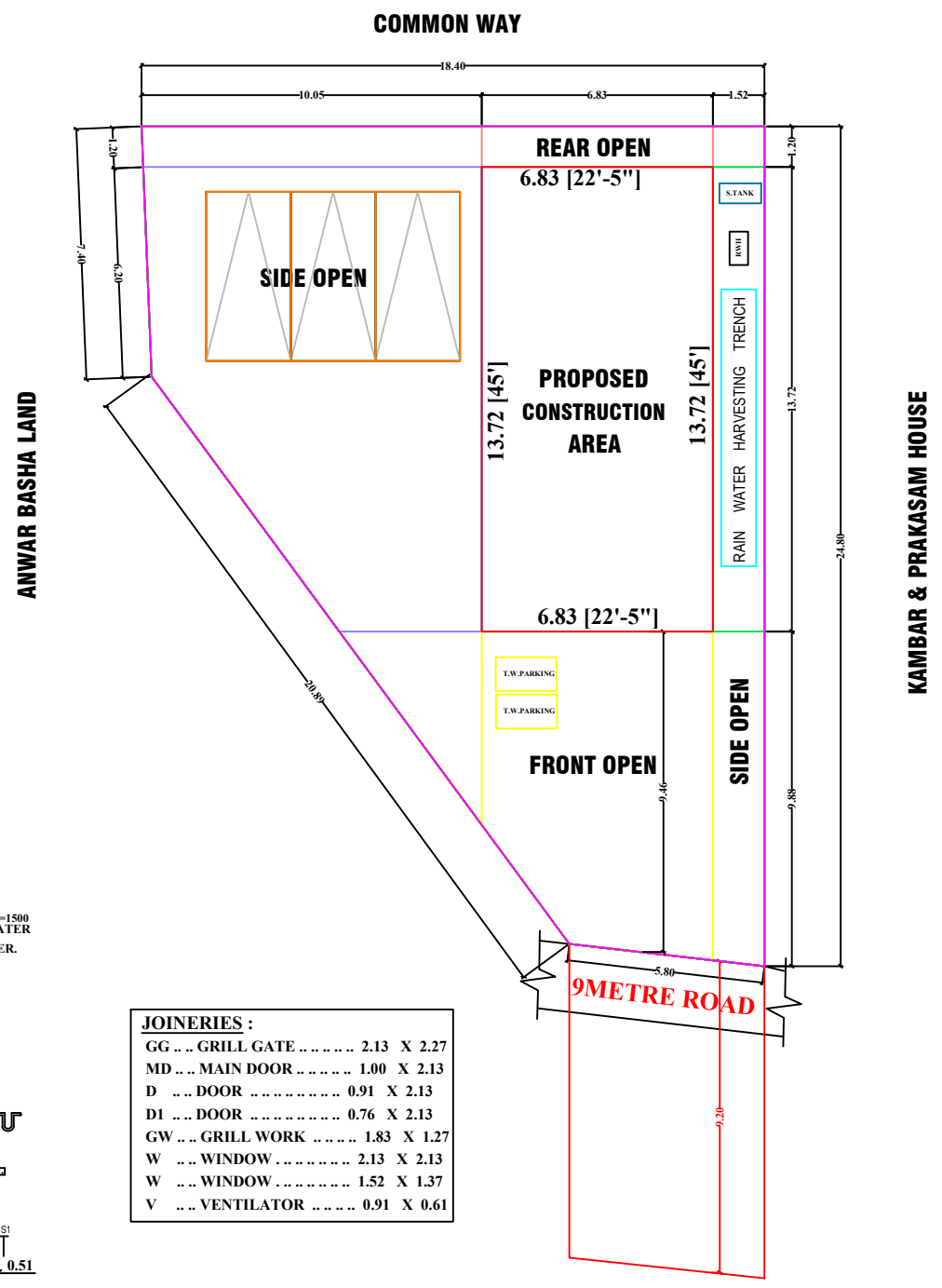
SITE PLAN-1:100
