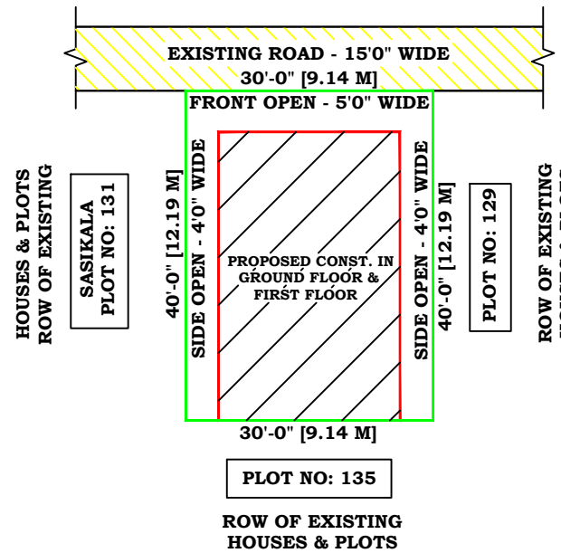
SITE PLAN:
