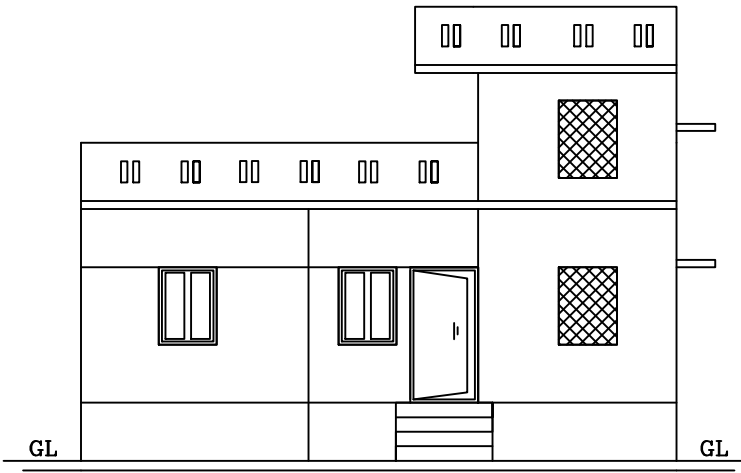
ELEVATION
