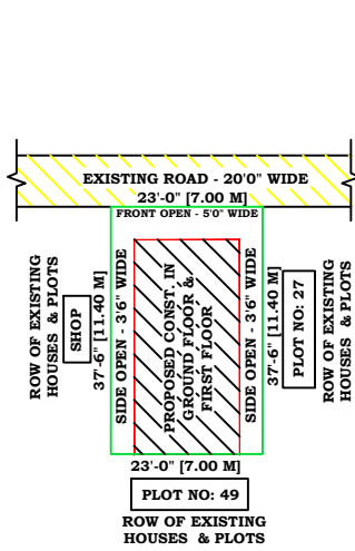
SITE PLAN:
