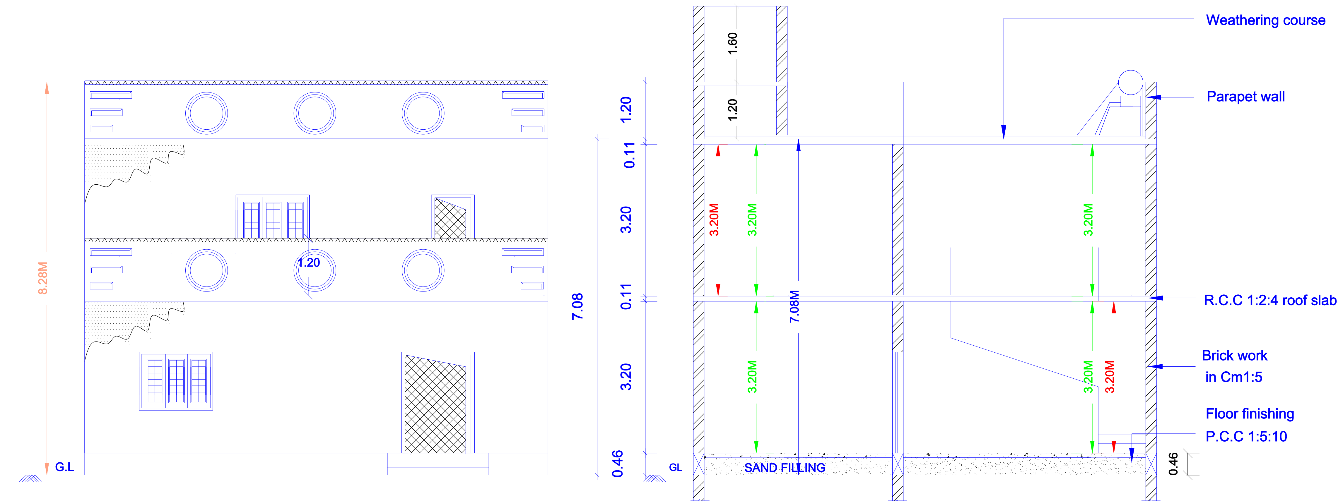
ELEVATION
