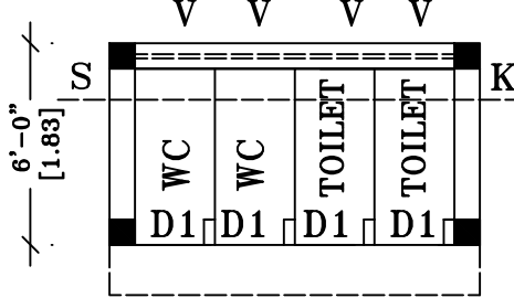
TOILET PLAN
