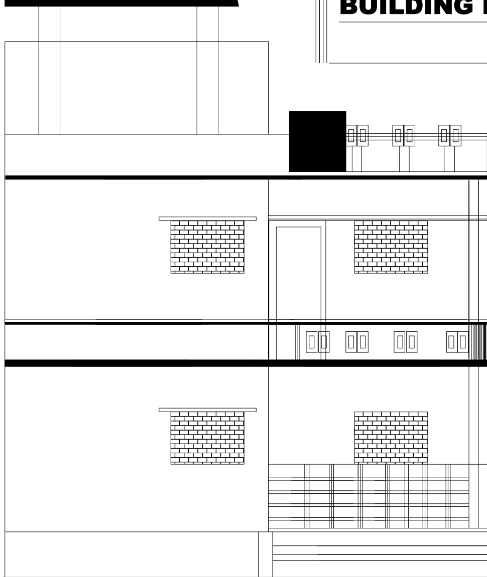
ELEVATION
