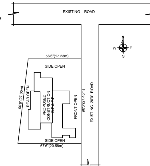
SITE PLAN:
