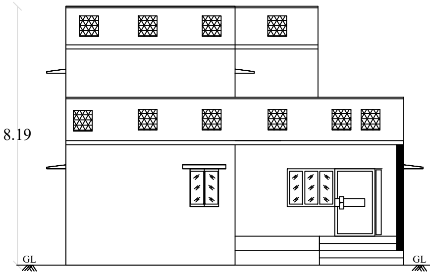
ELEVATION
