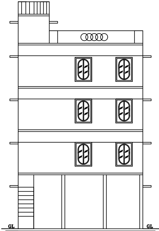
ELEVATION
