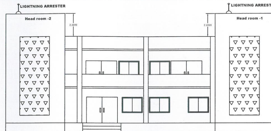
ELEVATION
