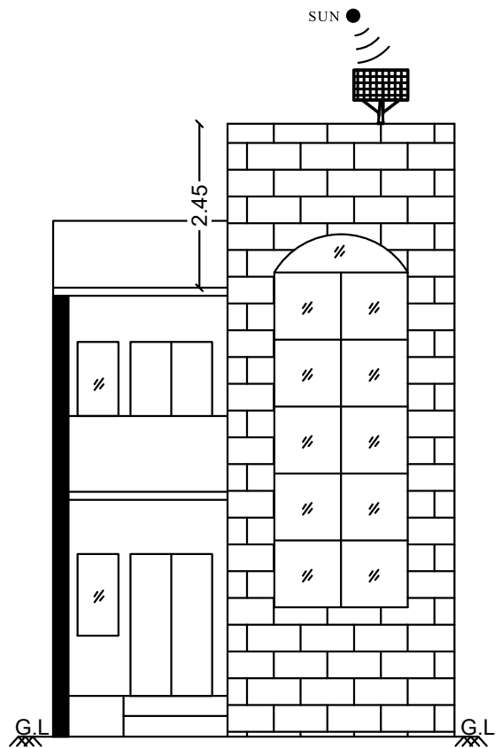
ELEVATION
