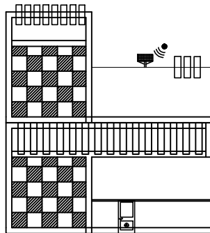
ELEVATION
