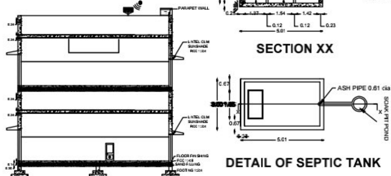
SECTION A-A
