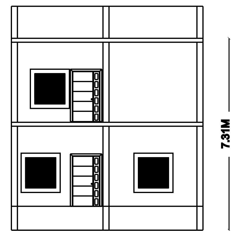
ELEVATION
