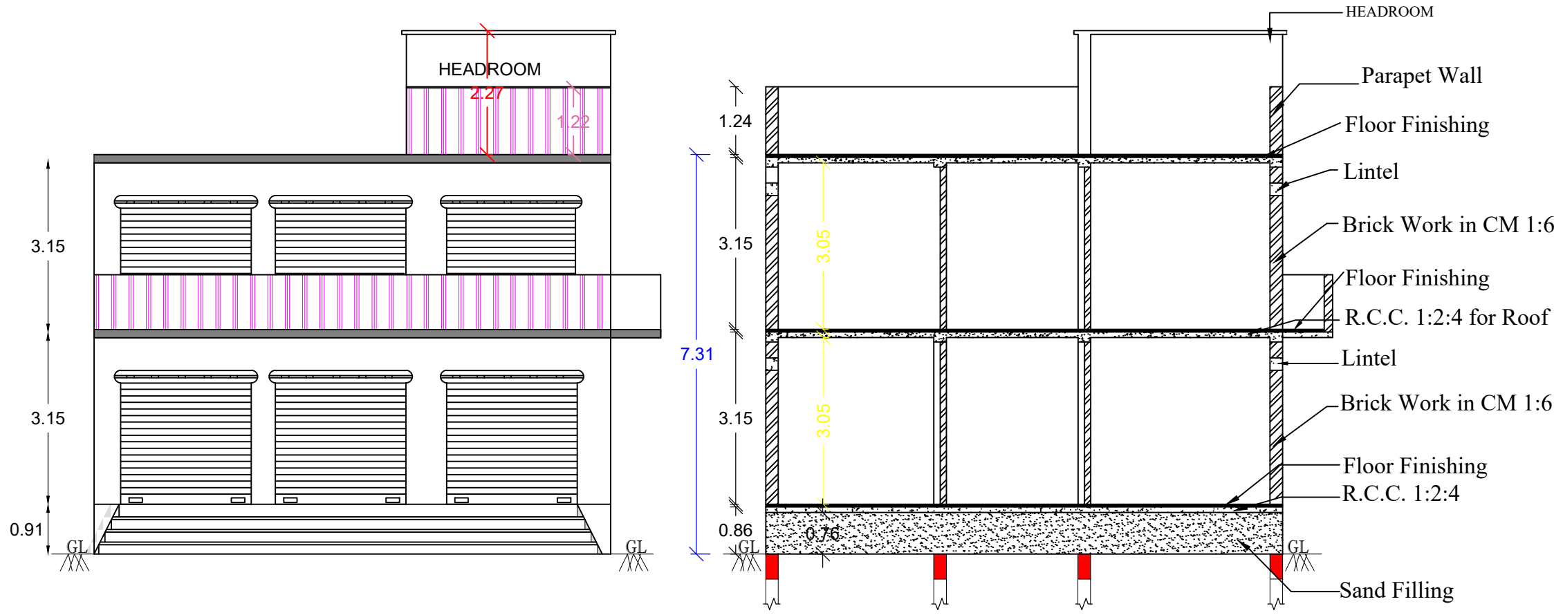
ELEVATION
