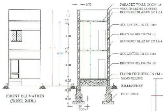
SECTION - AB
