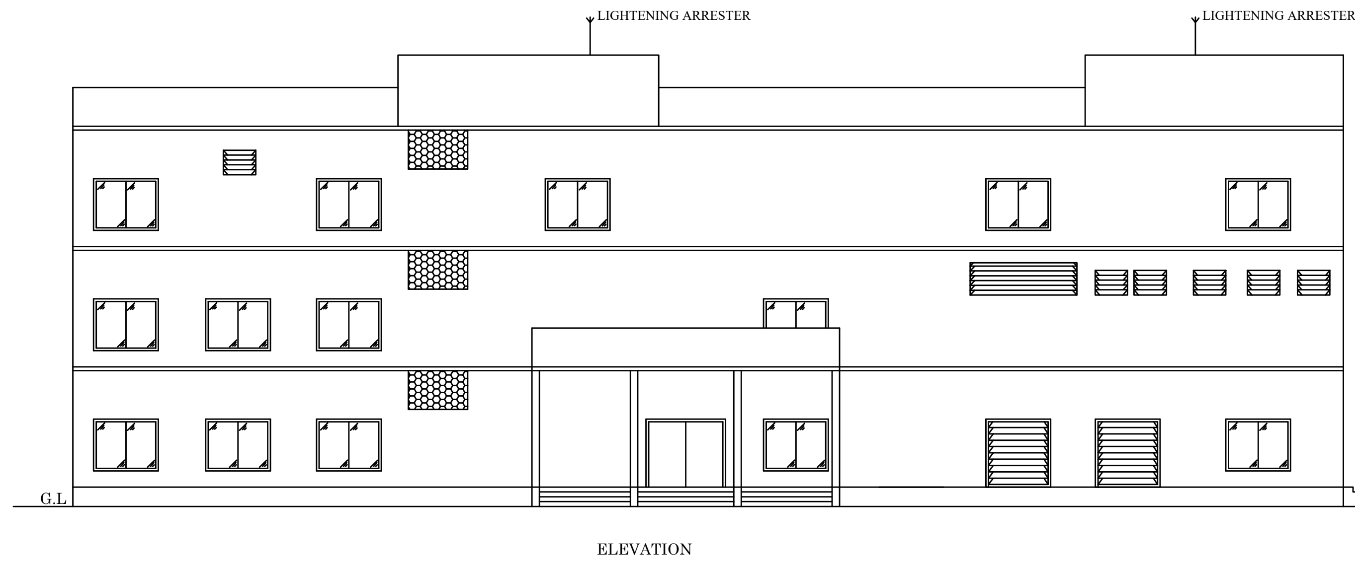
ELEVATION
