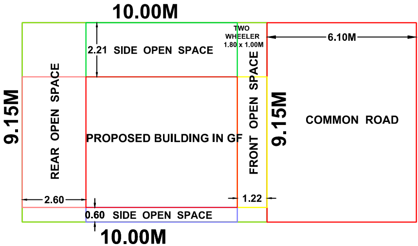
SITE PLAN SCALE : 1 :100
