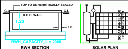
RWTH SECTION
