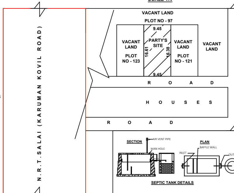
SITE PLAN SCALE 1:4
