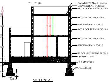
SECTION - AB
