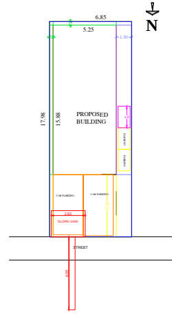
SITE PLAN - SCALE 1:100
