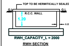
RWTH SECTION
