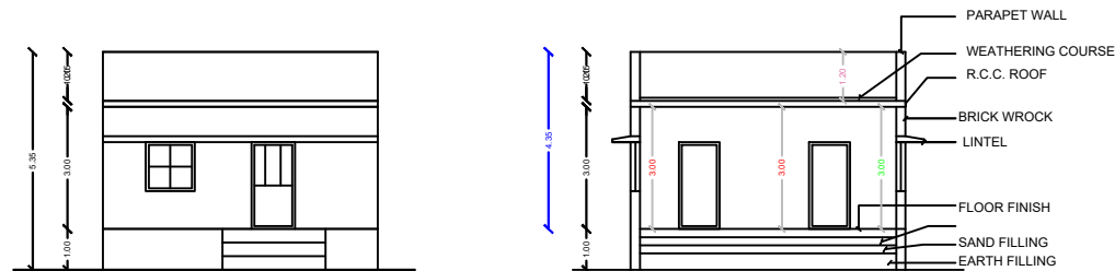
ELEVATION
