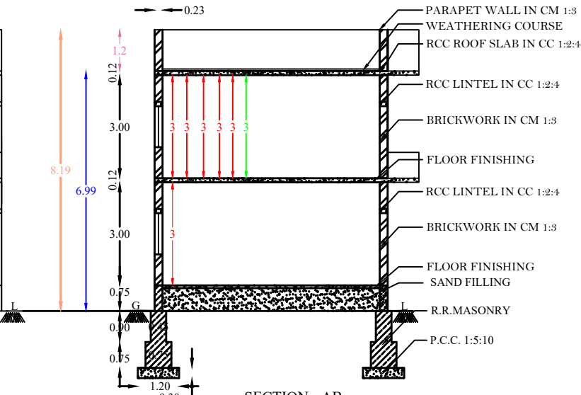
SECTION - AB
