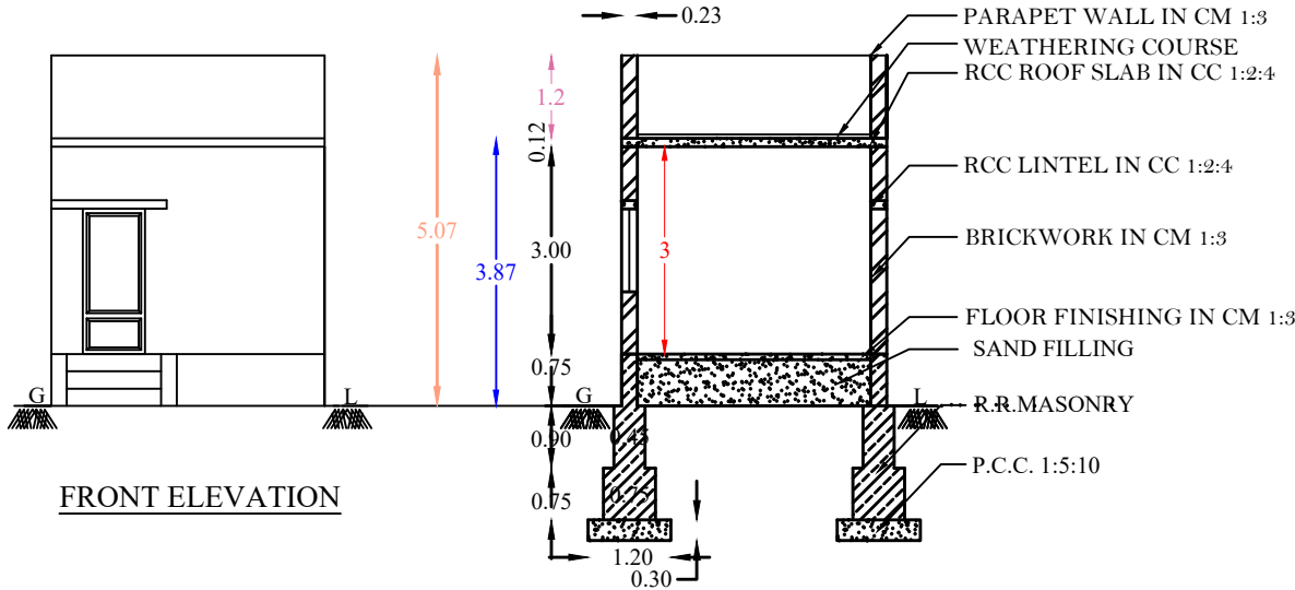
SECTION - AB
