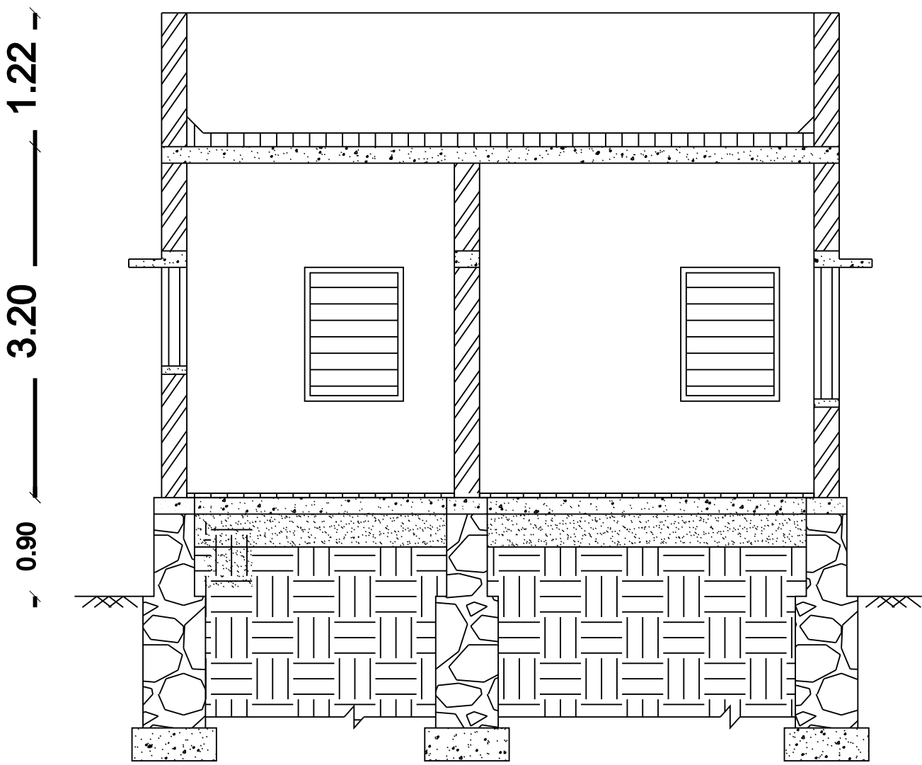
SECTION A-A
